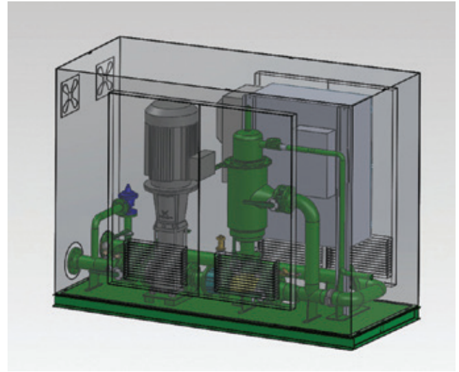
Vertical multietapa – 1 bomba mejorada – Se muestra la caja de aluminio De 5 a 50 HP; hasta 150 psi (10.3 bar); Hasta 500 gpm (31.5 l/s, 114 m³/h)
