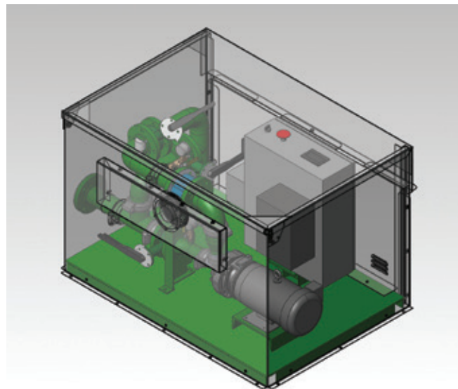
Succión de extremo horizontal; se muestra Serie LP De 5 a 10 HP; hasta 100 psi (6.9 bar); Hasta 200 gpm (12.6 l/s, 45.4 m³/h)
