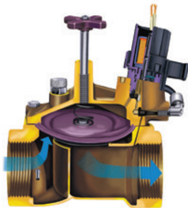
Vista transversal del modelo EFB-CP
