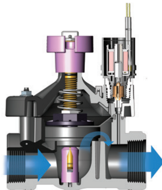
Vista transversal de una válvula PESB-R
